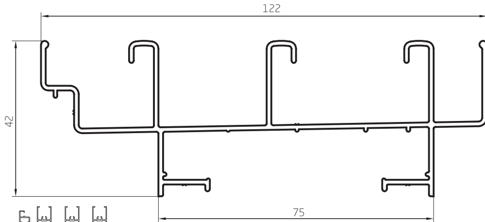
Marco Corredizo 3 Guías 1,158 kg/m 00095 Barras de 6,05m 4 Barras por Paquete
