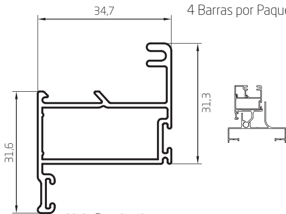
Hoja Banderola 0,537 kg/m 00187 Barras de 6,05m 6 Barras por Paquete
