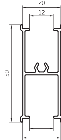
Travesaño Vertical 0,435 kg/m 00122
