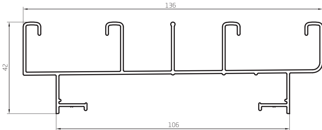
Marco Corredizo 4 Guías 1,259 kg/m 00096 Barras de 6,05m 4 Barras por Paquete
