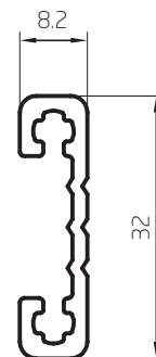
Toallero 0,301 kg/m 00555 Barras de 6,05m 10 Barras por Paquete
