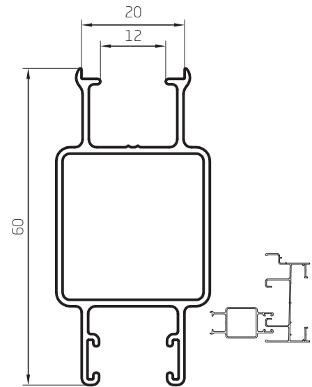
Parante Lateral Ventana Balcón 0,633 kg/m 00123 Barras de 6,20m 6 Barras por Paquete
