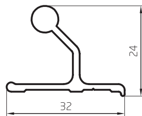
Bisagra 0,355 kg/m 00186 Barras de 6,05m 10 Barras por Paquete
