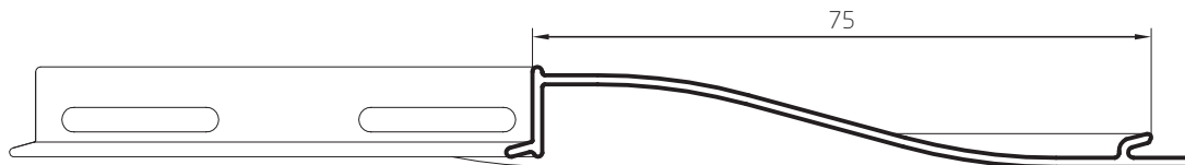
Tablilla Curva Postigón 75mm troquelada (13 tablillas / metro lineal) 0,290 kg/m 00427 Barras de 6,05m 15 Barras por Paquete
