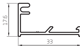
Porta Contravidrio 0,234 kg/m 00128 Barras de 6,05m 12 Barras por Paquete
