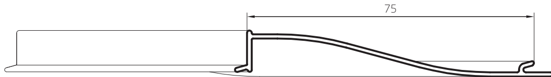
Tablilla Curva Postigón 75mm (13 tablillas / metro lineal) 0,290 kg/m 00417 Barras de 6,05m 15 Barras por Paquete
