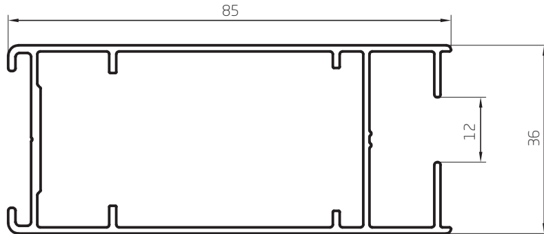
Parante Puerta F 85mm 0,975 kg/m 00178 Barras de 6,20m 4 Barras por Paquete
