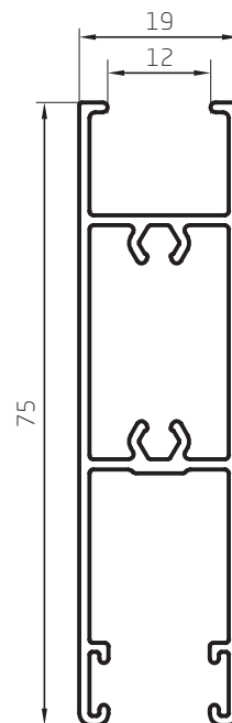
Travesaño 75mm 0,750 kg/m 00113
