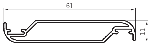
Tablilla Giratoria 0,457 kg/m 00414 Barras de 6,05m 10 Barras por Paquete
