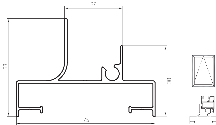
Marco Ventiluz 0,779 kg/m 00184 Barras de 6,05m 4 Barras por Paquete
