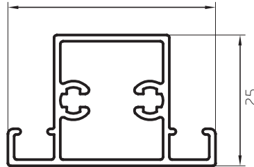
Travesaño Puerta Mosquitero 0,501 kg/m 00120 Barras de 6,05m 9 Barras por Paquete
