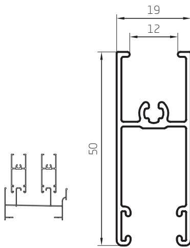
Travesaño Ventana Corrediza Reforzado 0,509 kg/m 09002
