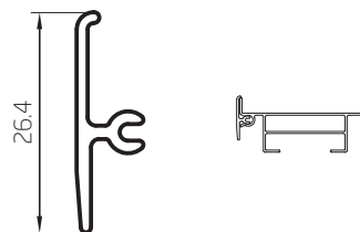
Tapajunta 0,149 kg/m 00145 Barras de 6,05m 20 Barras por Paquete
