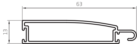
Zócalo Cortina de Enrollar 0,485 kg/m 00416 Barras de 6,05m 8 Barras por Paquete
