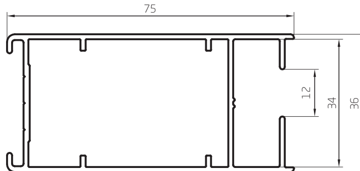
Parante Puerta F 75mm 0,990 kg/m 00179 Barras de 6,20m 4 Barras por Paquete
