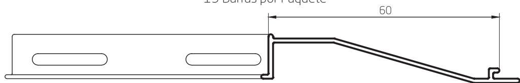
Tablilla Postigón 60mm troquelada (15 tablillas / metro lineal) 0,248 kg/m 00430 Barras de 6,05m 15 Barras por Paquete
