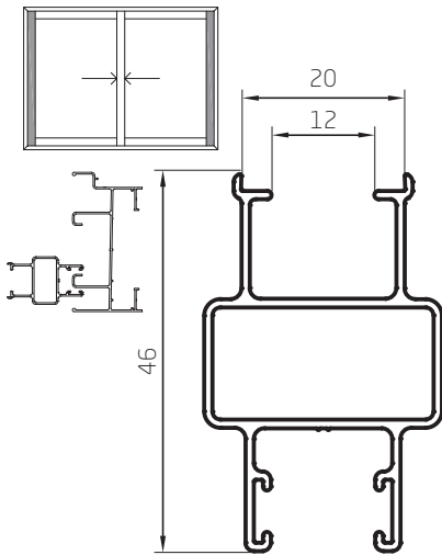
Parante Lateral 0,453 kg/m 00103 Barras de 6,05m 10 Barras por Paquete
