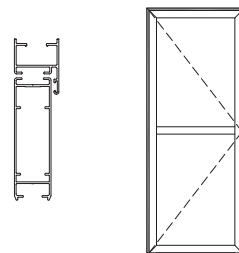
Marco Angosto 30mm 0,408 kg/m 00165 Barras de 6,05m 10 Barras por Paquete
