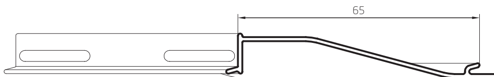
Tablilla Postigón 65mm troquelada (15 tablillas / metro lineal) 0,250 kg/m 00428 Barras de 6,05m 15 Barras por Paquete
