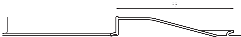
Tablilla Postigón 65mm (15 tablillas / metro lineal) 0,250 kg/m 00418 Barras de 6,05m 15 Barras por Paquete
