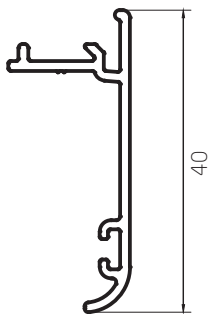
Tapajuntas Recto 0,251 kg/m 09011 Barras de 6,05m 18 Barras por Paquete
