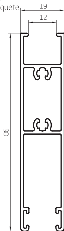
Travesaño 86mm 0,929 kg/m 00127
