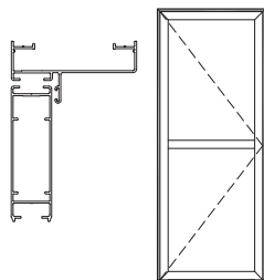
Marco 75mm Interior/Exterior 0,615 kg/m 00152 Barras de 6,20m 6 Barras por Paquete
