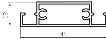
Travesaño 0,388 kg/m 00115 Barras de 6,05m 10 Barras por Paquete
