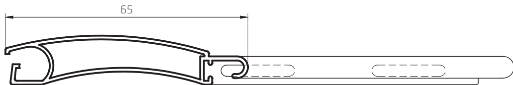
Tablilla Cortina de Enrollar troquelada 0,426 kg/m 00433 Barras de 6,05m 10 Barras por Paquete
