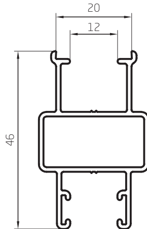
Parante Lateral 0,510 kg/m 09003 Barras de 6,05m 10 Barras por Paquete
