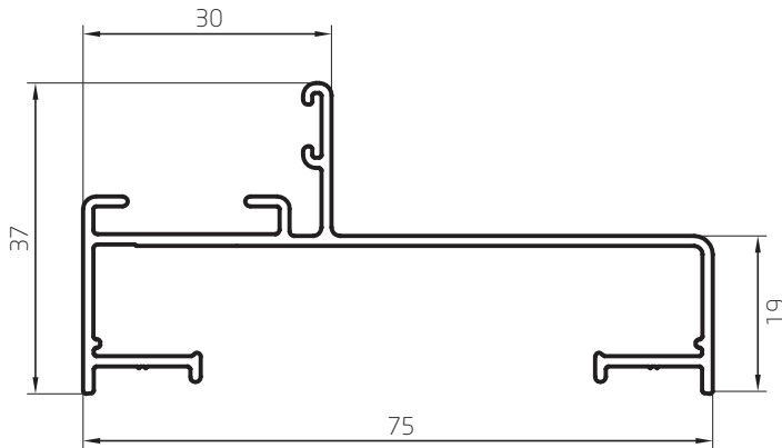
Marco 75mm Interior/Exterior 0,615 kg/m 00152 Barras de 6,20m 6 Barras por Paquete
