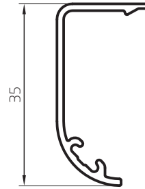
Tapajuntas 0,250 kg/m 02826 Barras de 6,05m 18 Barras por Paquete
