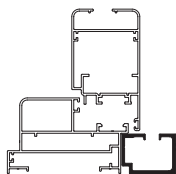
Guía Inferior Marco Puerta Libro 0,580 kg/m 02871 Barras de 6,05m 6 Barras por Paquete
