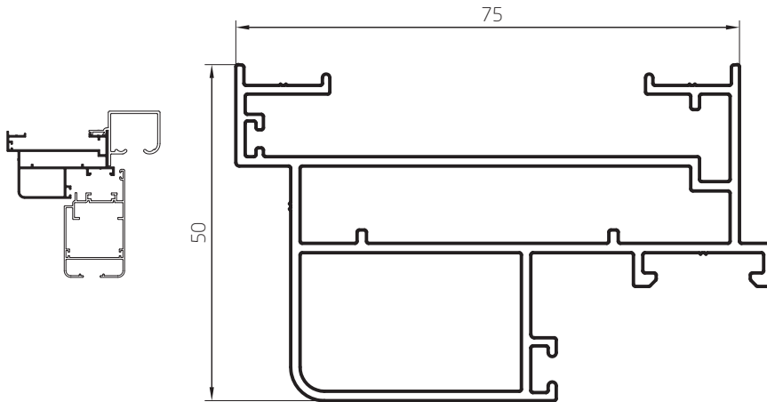
Marco Puerta Libro 1,292 kg/m 02870 Barras de 6,20m 4 Barras por Paquete
