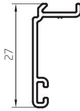
Tapajuntas 0,148 kg/m 09013 Barras de 6,05m 18 Barras por Paquete
