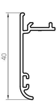
S Tapajuntas Recto 0,251 kg/m 09011 Barras de 6,05m 18 Barras por Paquete
