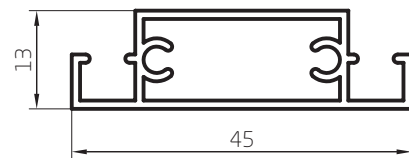
Travesaño 0,388 kg/m 00115 Barras de 6,05m 10 Barras por Paquete
