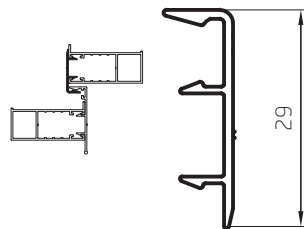
Encuentro Central Exterior 0,154 kg/m 02813 Barras de 6,05m
