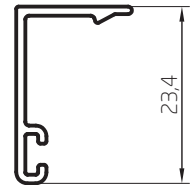
Tapajuntas 0,148 kg/m 02892 Barras de 6,05m 18 Barras por
